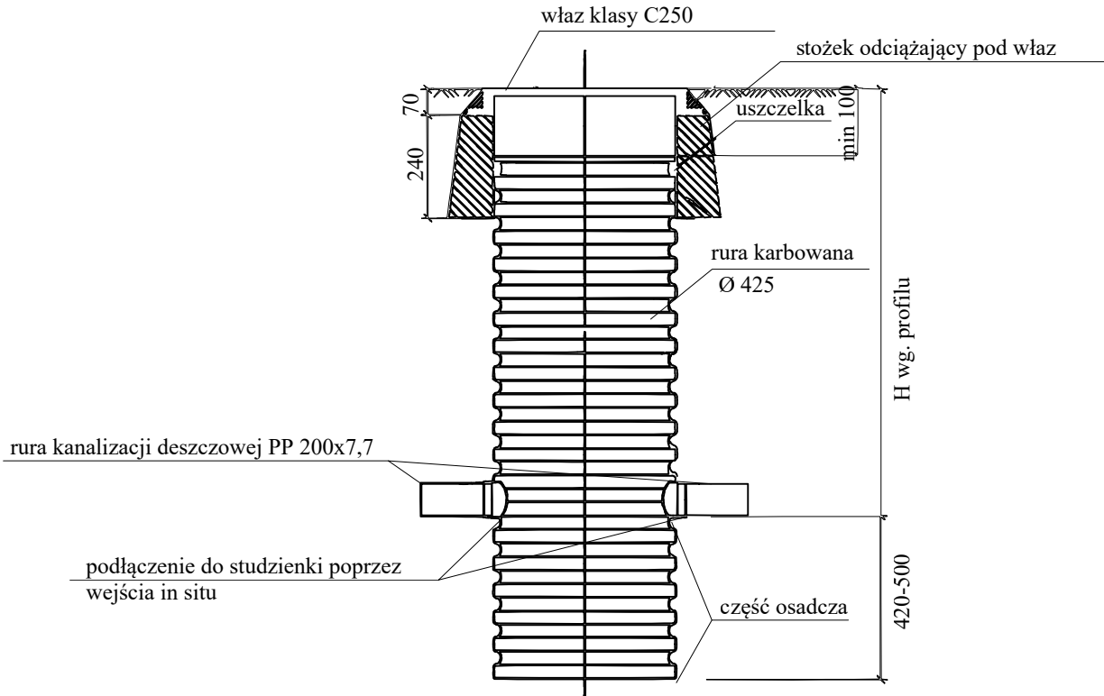
schemat studni rewizyjnej Ø425
