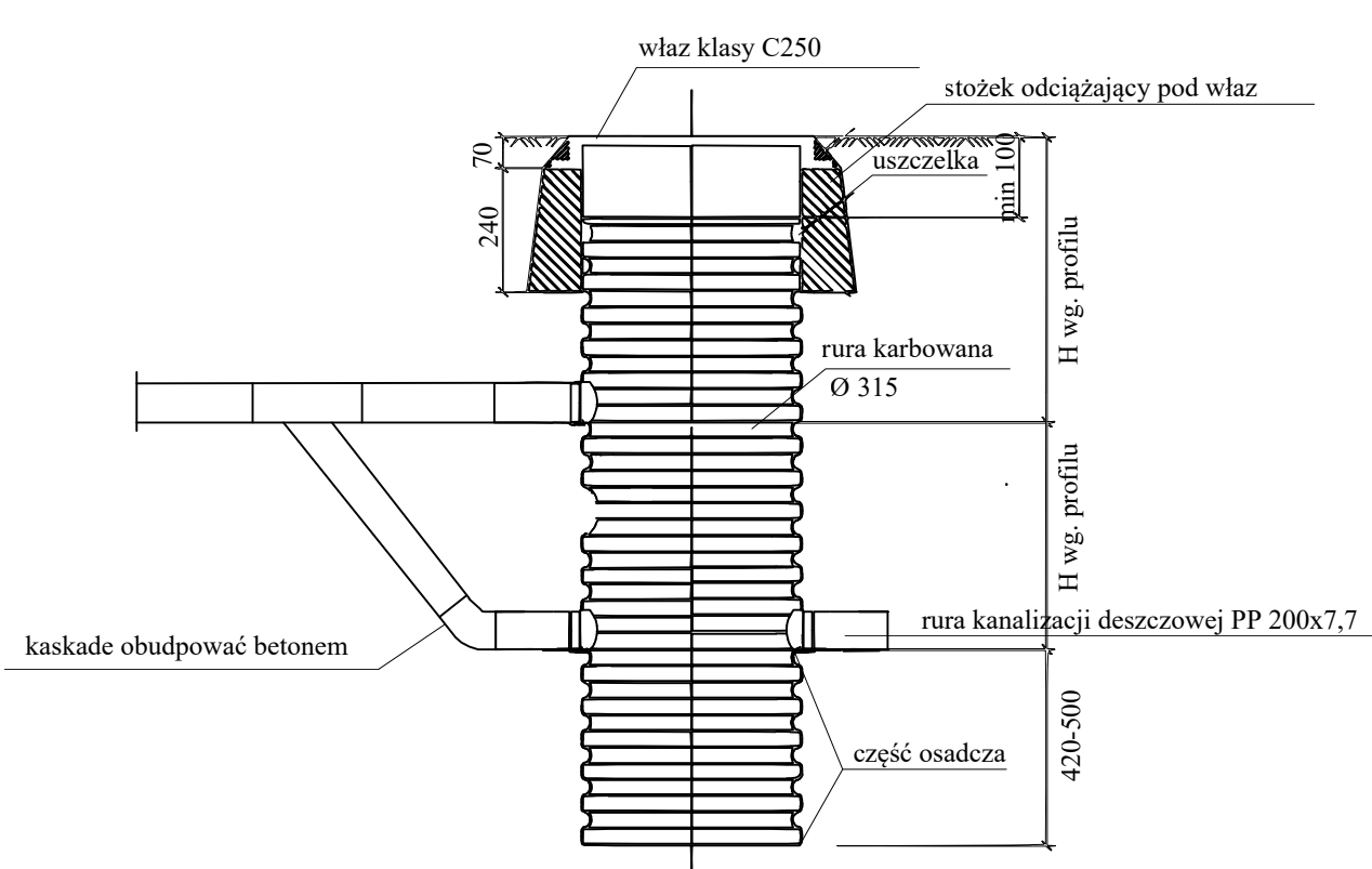
schemat studzienki drenarskiej zbiorczej kaskadowej Ø315
